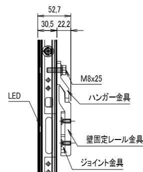
壁掛け金具 A部詳細図 1/5
