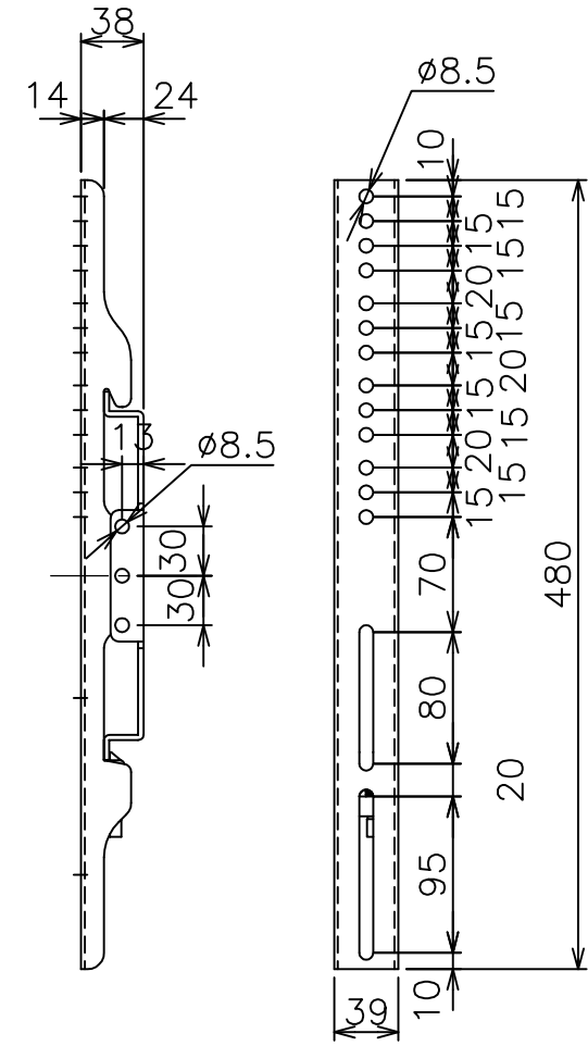
アタッチメント穴位置図
