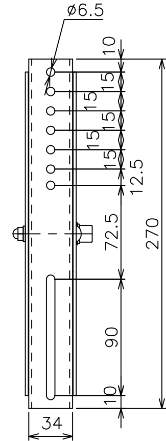
アタッチメント穴位置図
