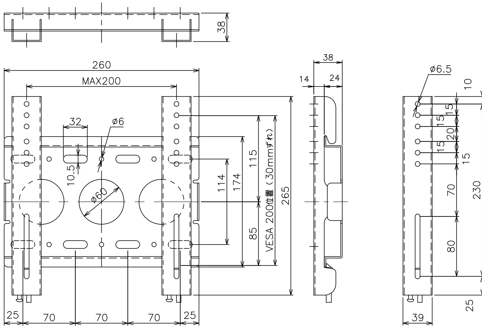
アタッチメント穴位置図
