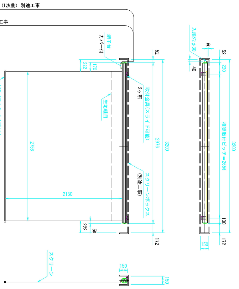
外観図 S=1/30
