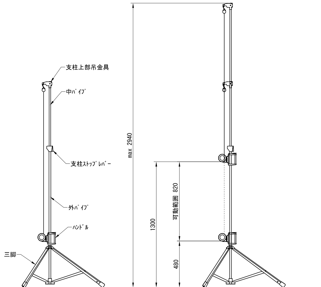
脚収納図
