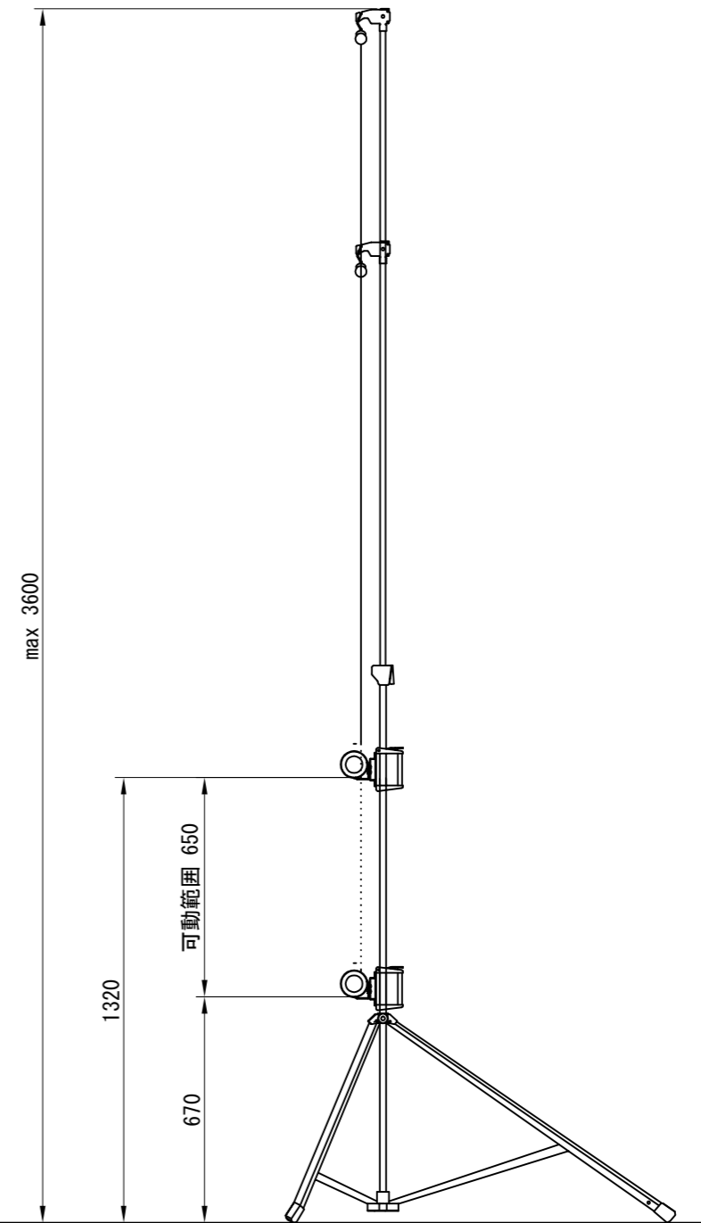
脚収納図
