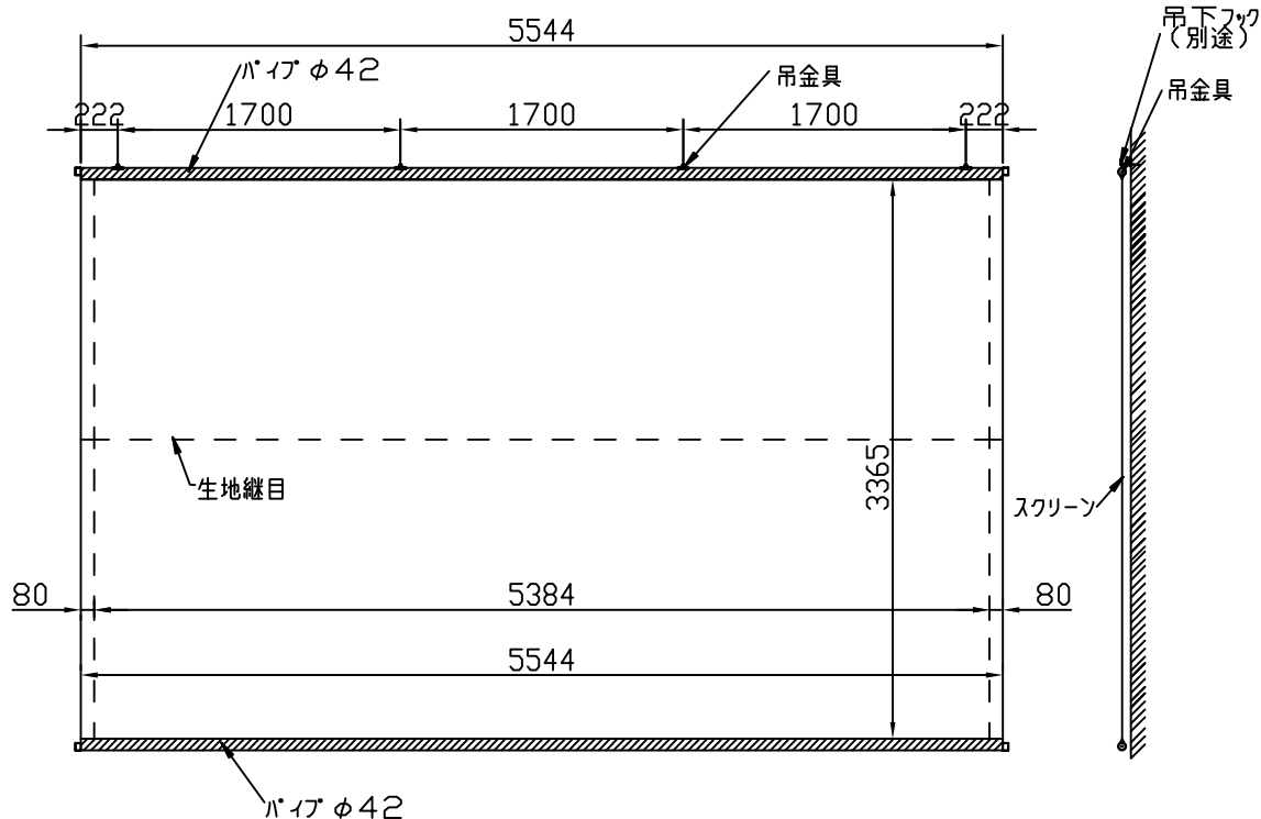
外觀図 1/50
