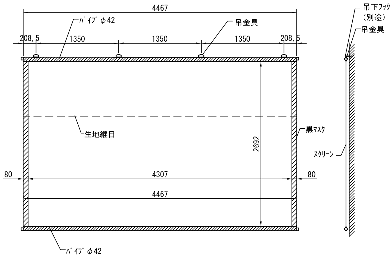
外観図 1/40
