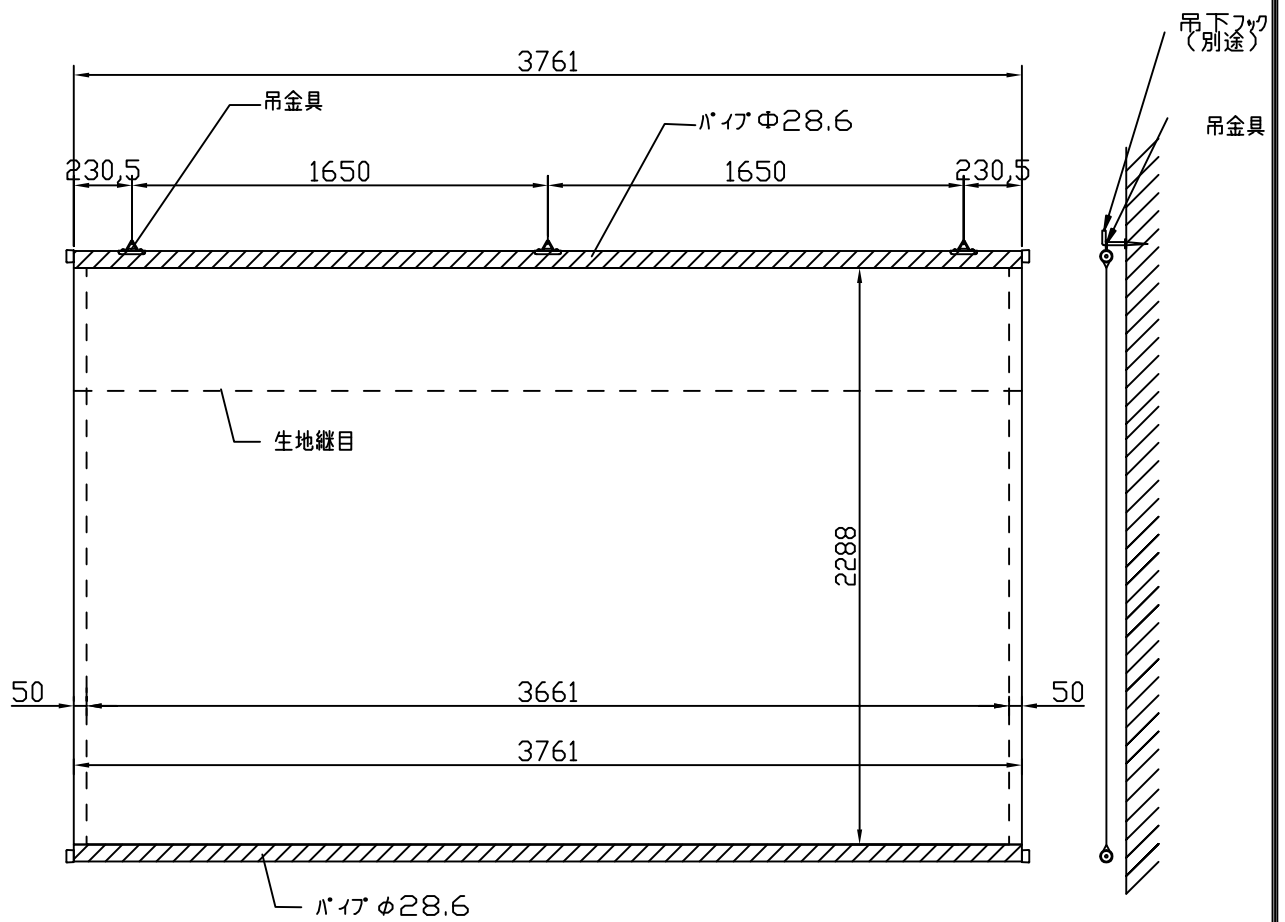
外観図1/30
