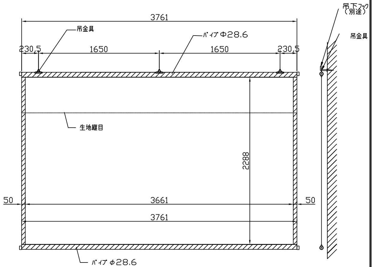
外観図1/30
