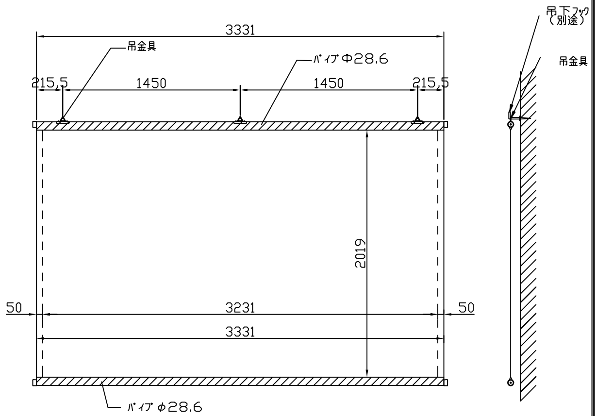
外観図1/30
