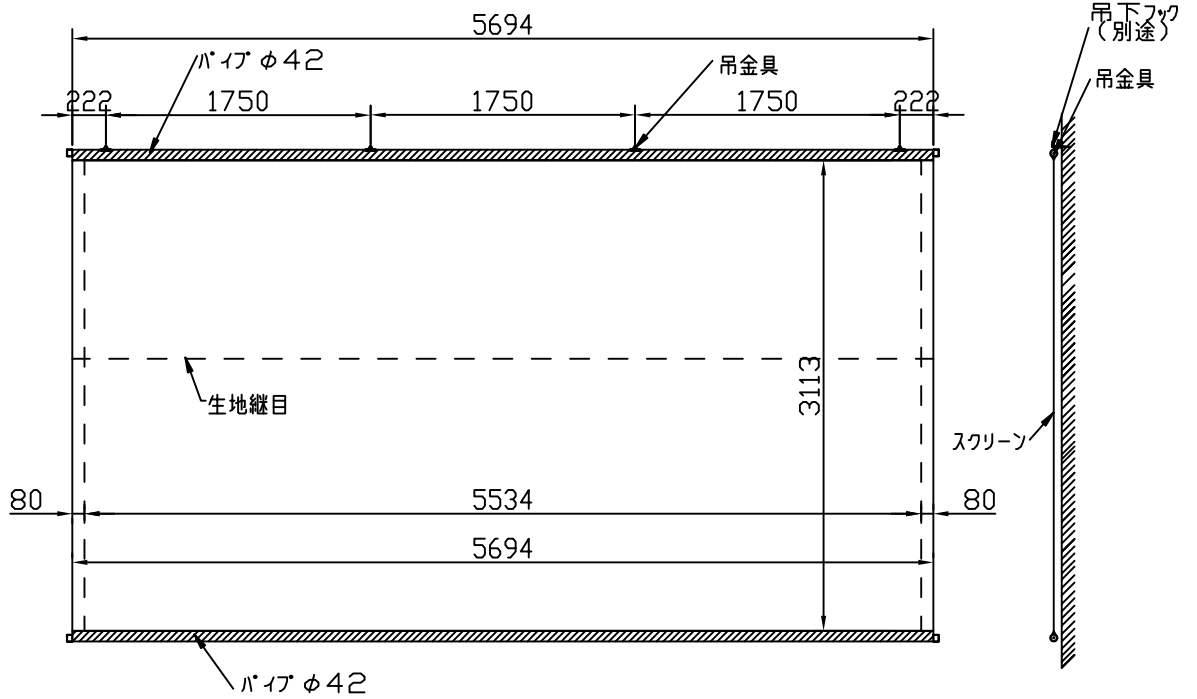
断面図 1/50
