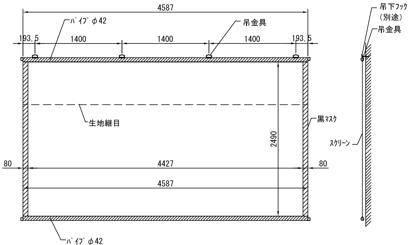
外観図 1/40
