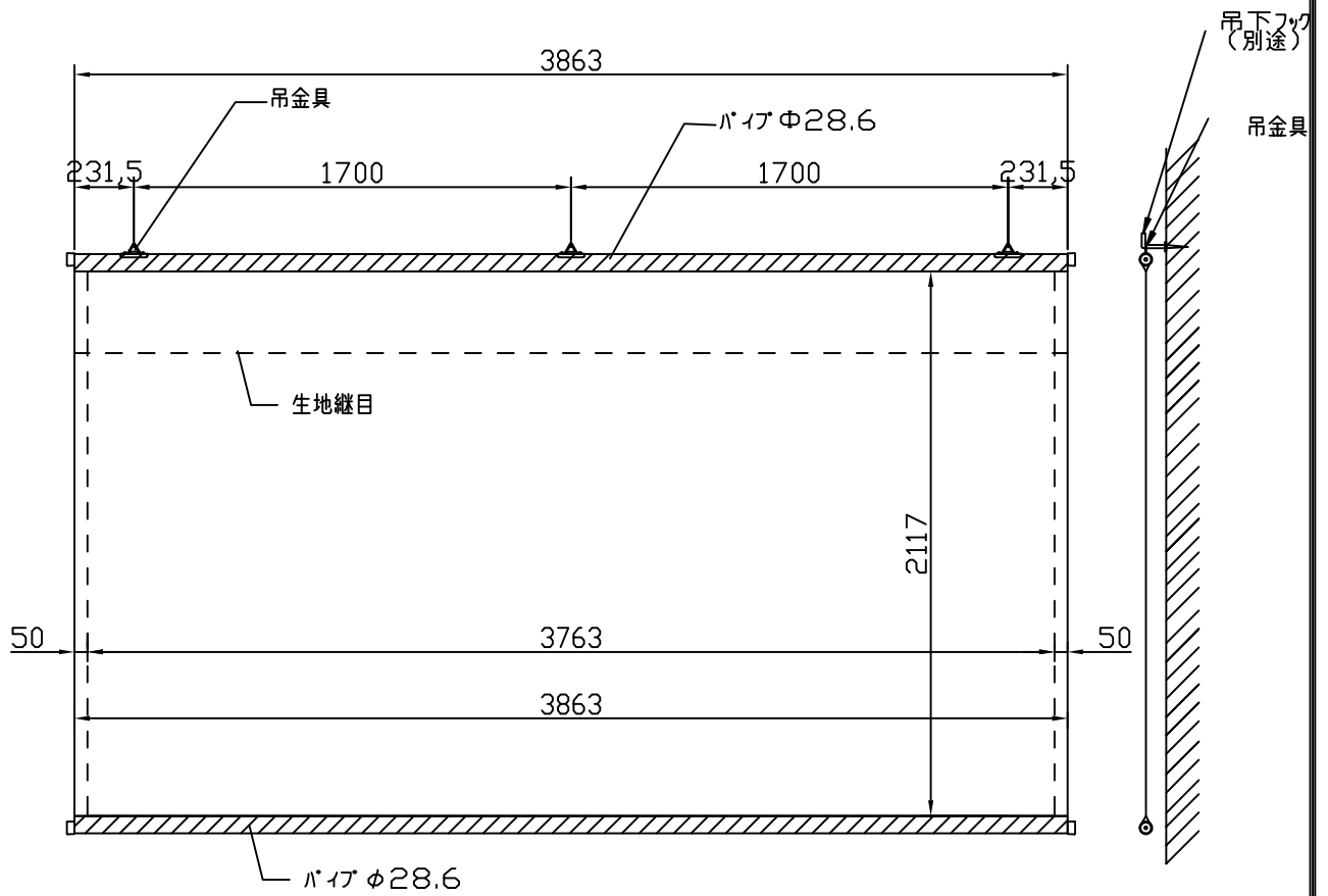
外観図1/30
