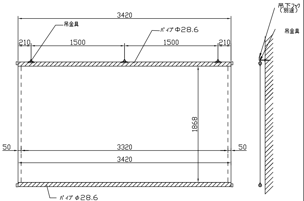
外観図1/30
