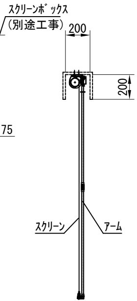
側面図 1/30
