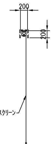
断面図 1/60
