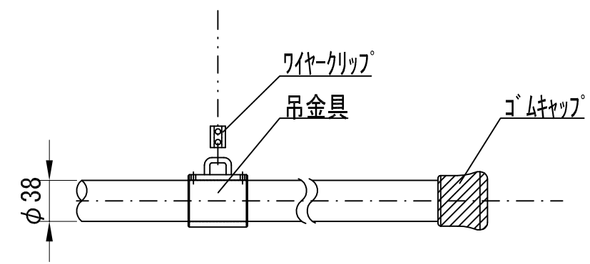
バトンパイφ詳細図 S=1/5
