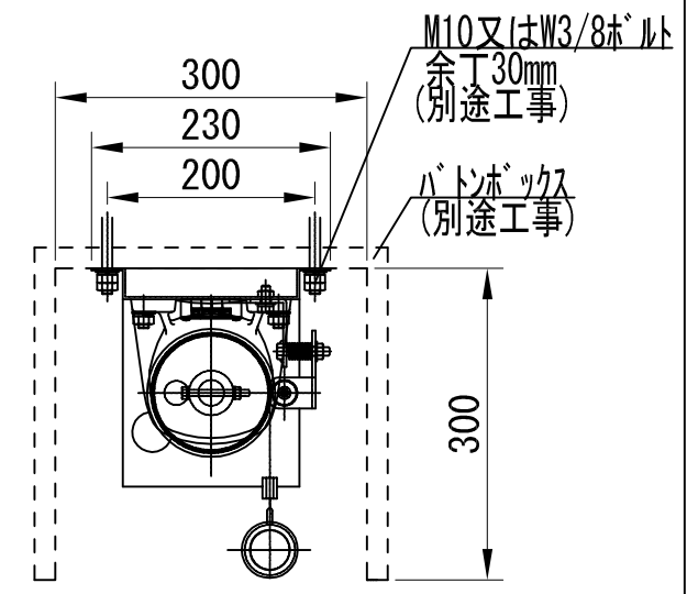
詳細図 S=1/8
