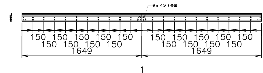
壁取付金具図
