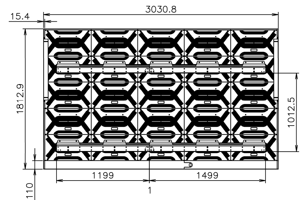
背面図
