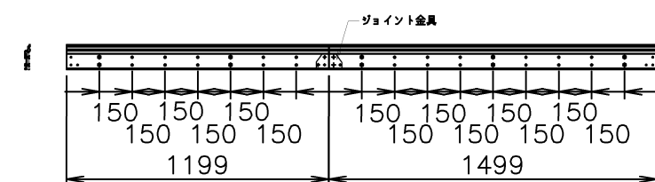
壁取付金具図
