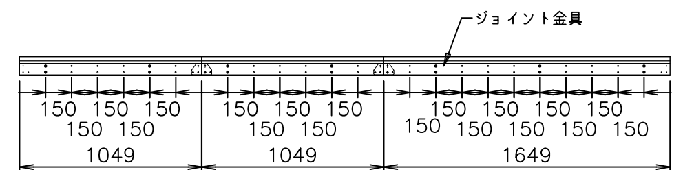
壁取付金具図
