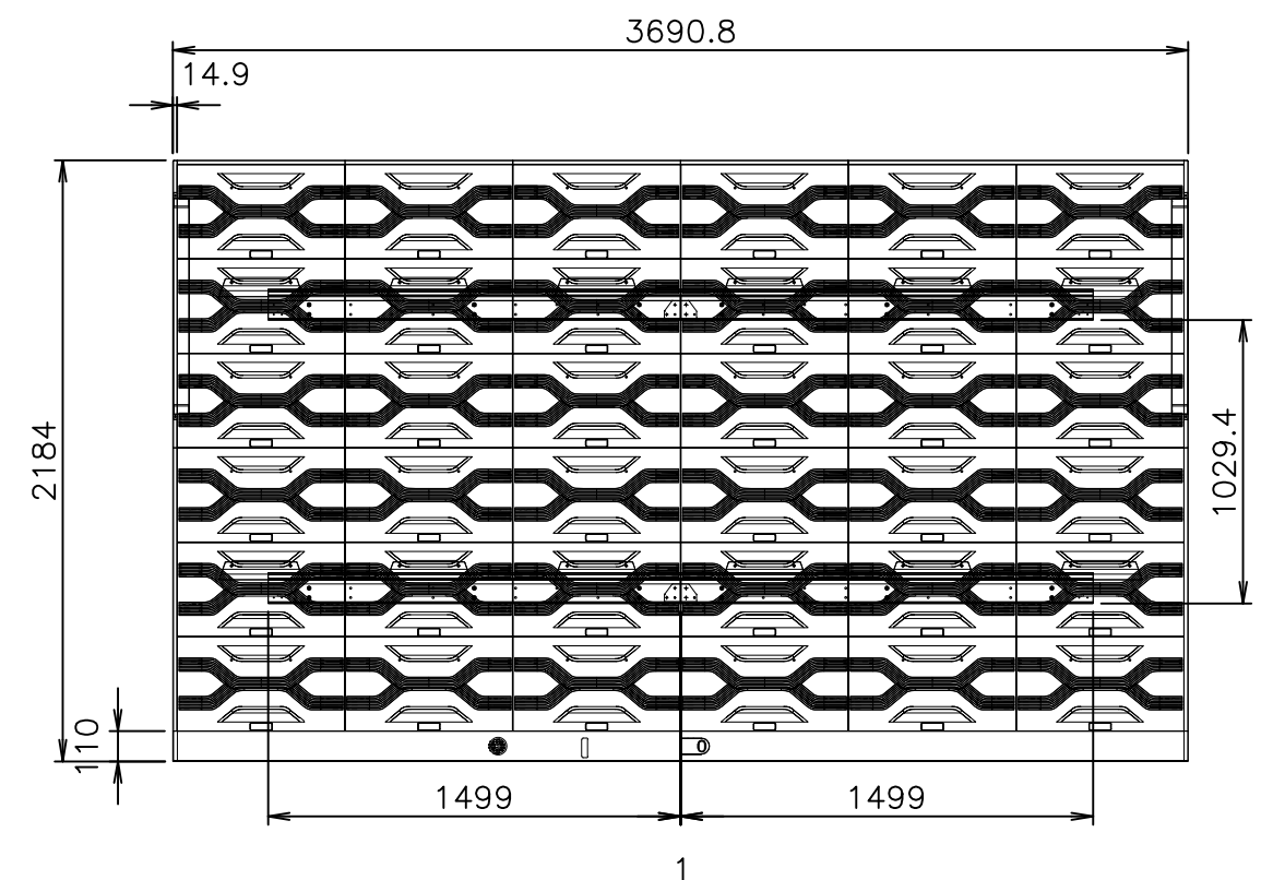
背面図
