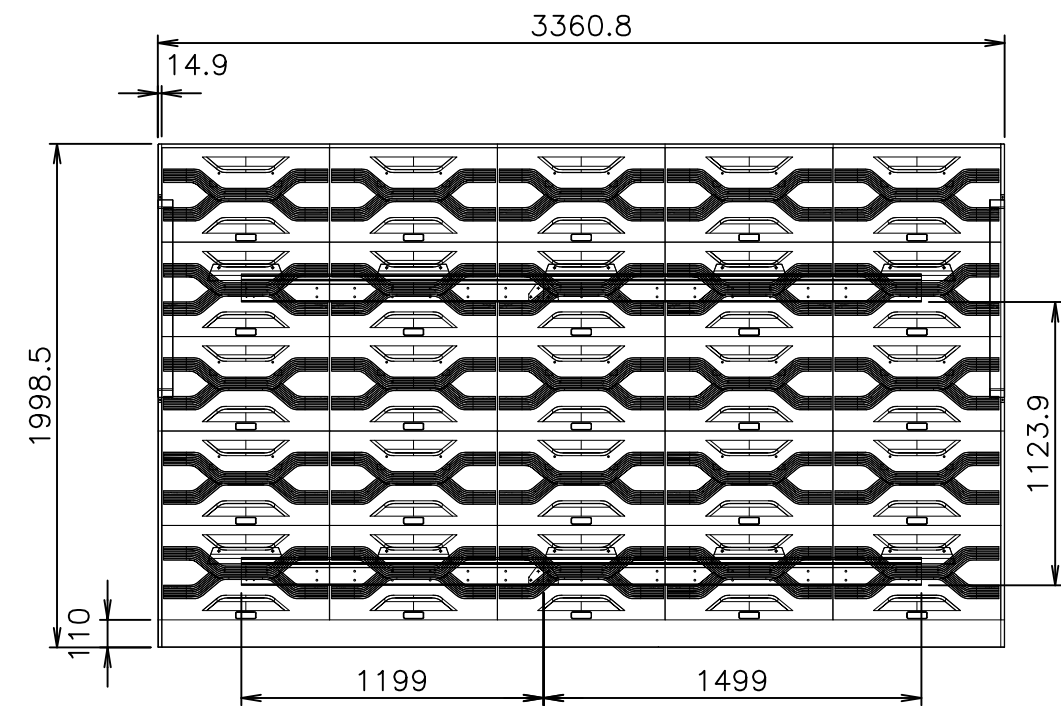
1 背面図
