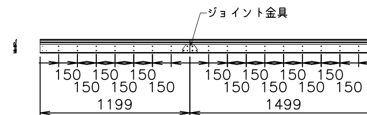
壁取付金具図
