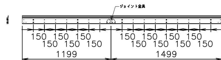
壁取付金具図
