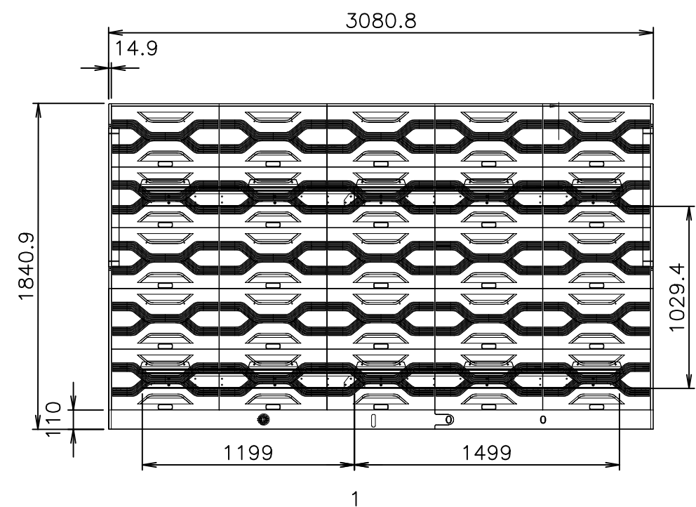
背面図
