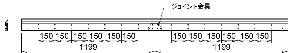
壁取付金具図
